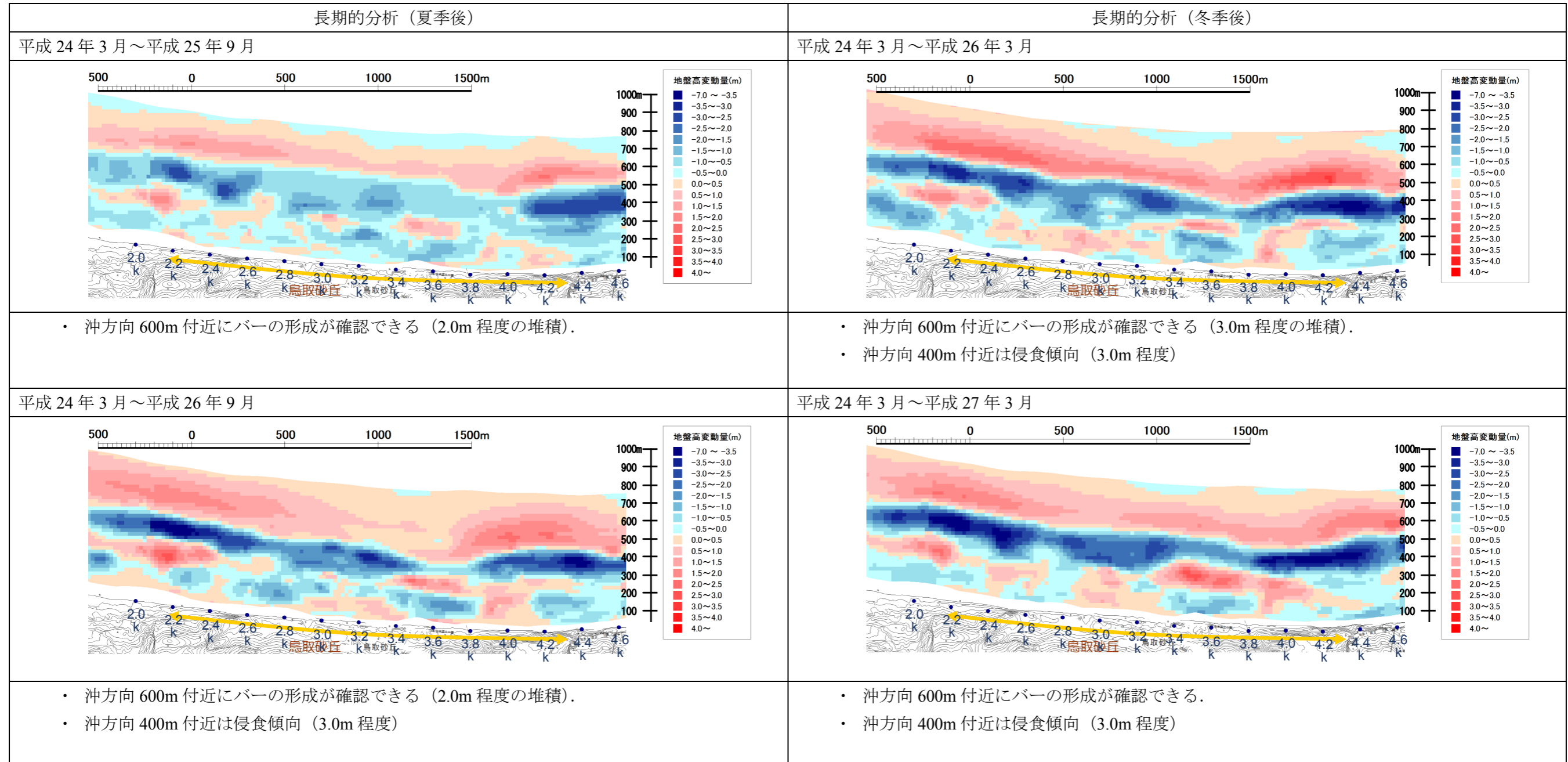
図 4.3.11 標高差分図(平成 24 年 3 月を基準とした長期的分析)
