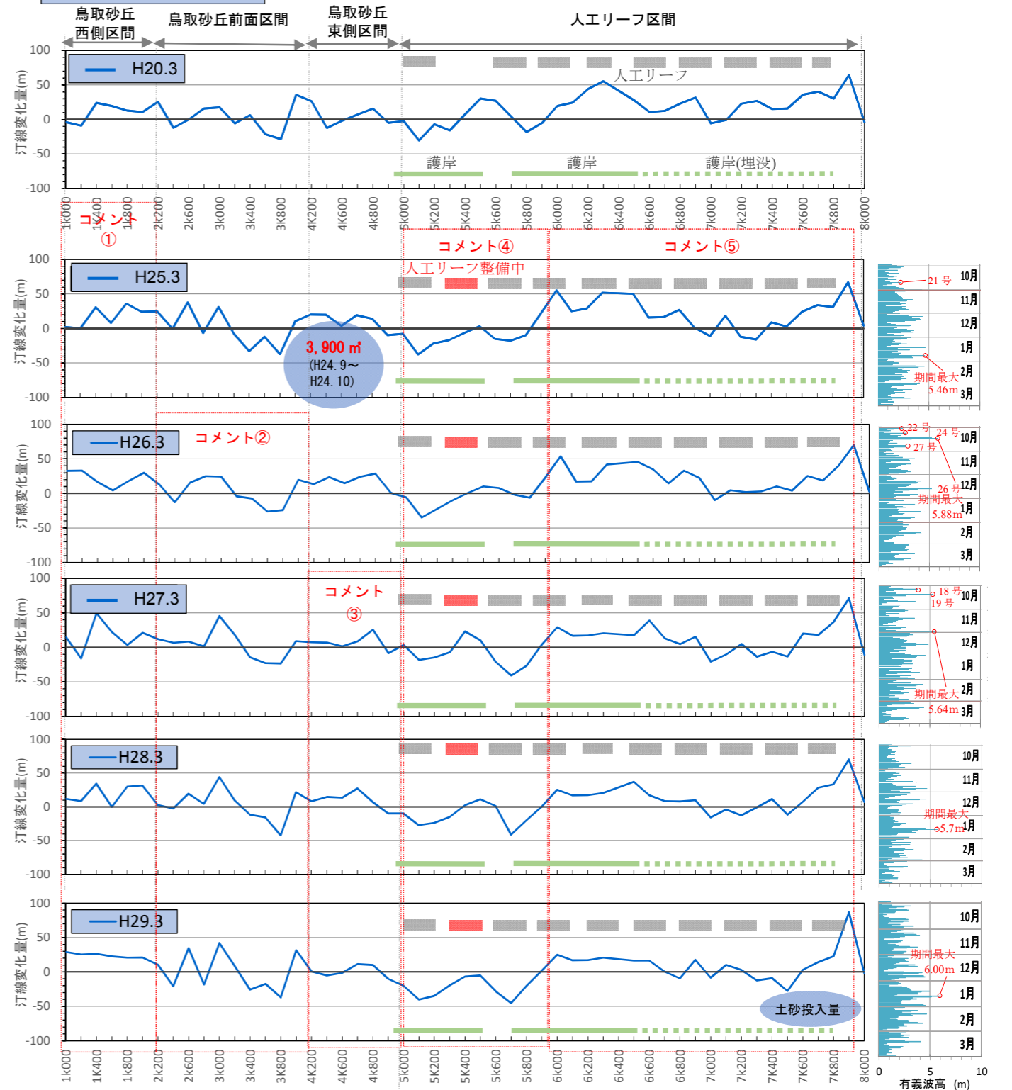
図 4.3.5 サンドリサイクル開始以後の汀線変化状況図(平成 18 年 3 月基準)
