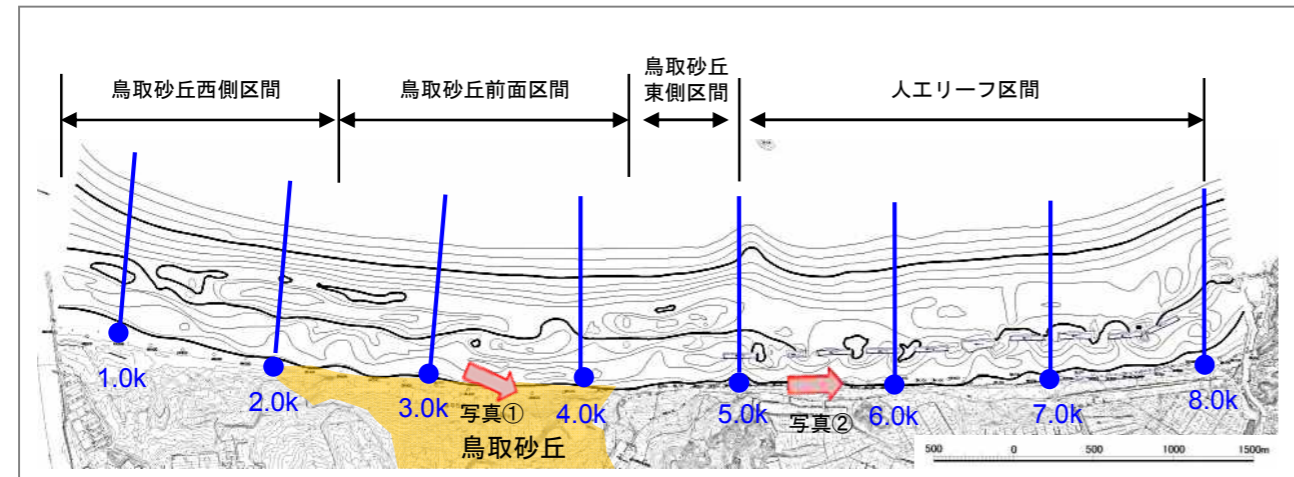
図 4.3.1 区間別の代表測線位置図(等深線図 H29.3 測量)
