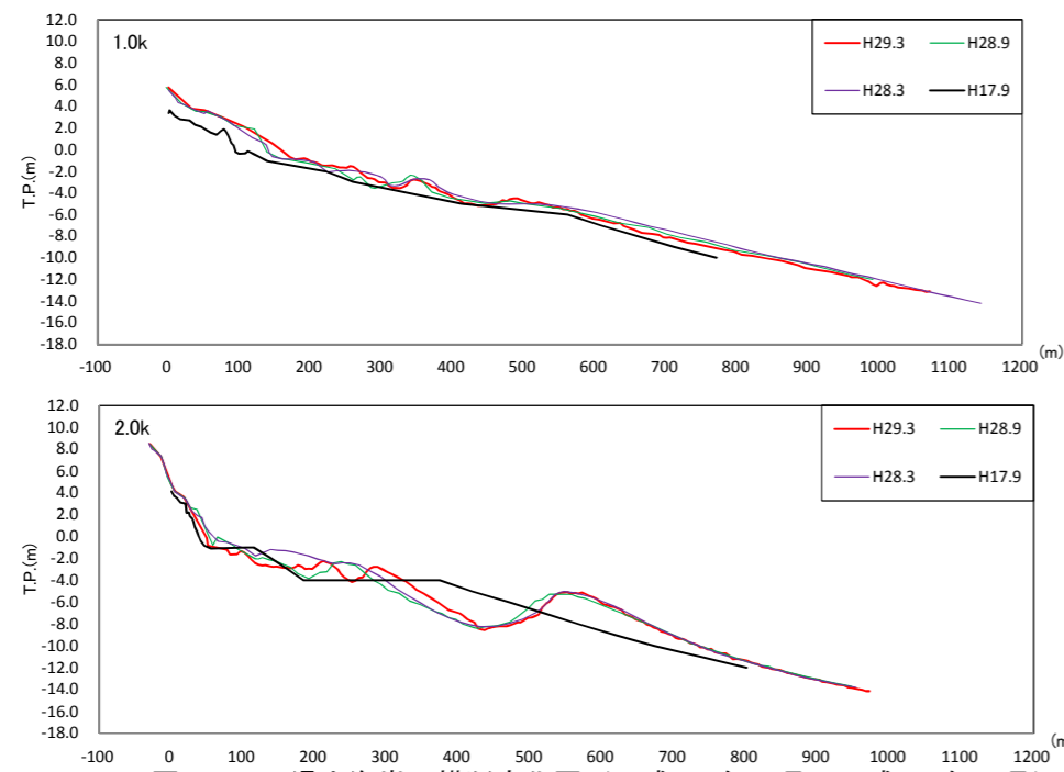
図 4.3.9 湯山海岸の横断変化図（平成 17 年 9 月～平成 29 年 3 月）(1)
