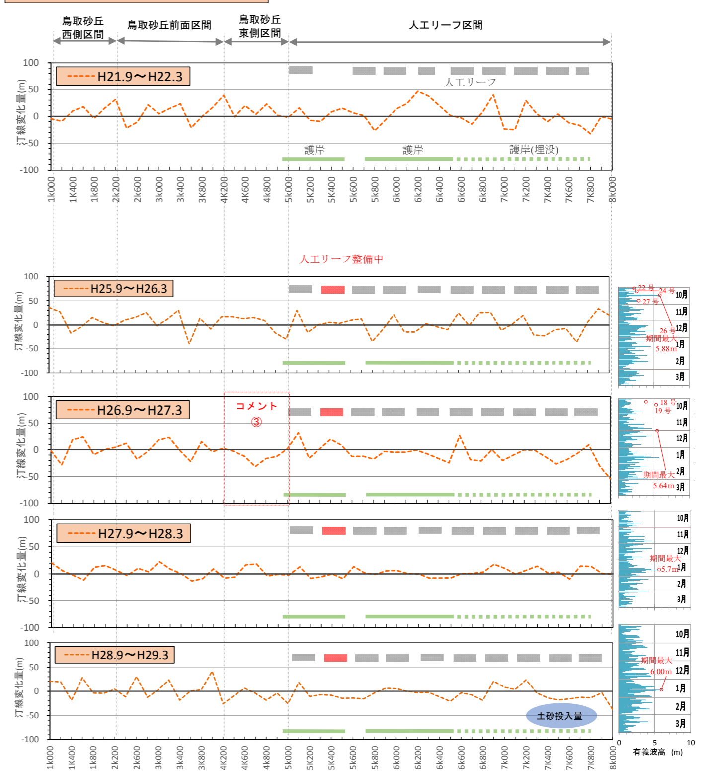
図 4.3.7 サンドリサイクル開始以後の汀線変化状況図
