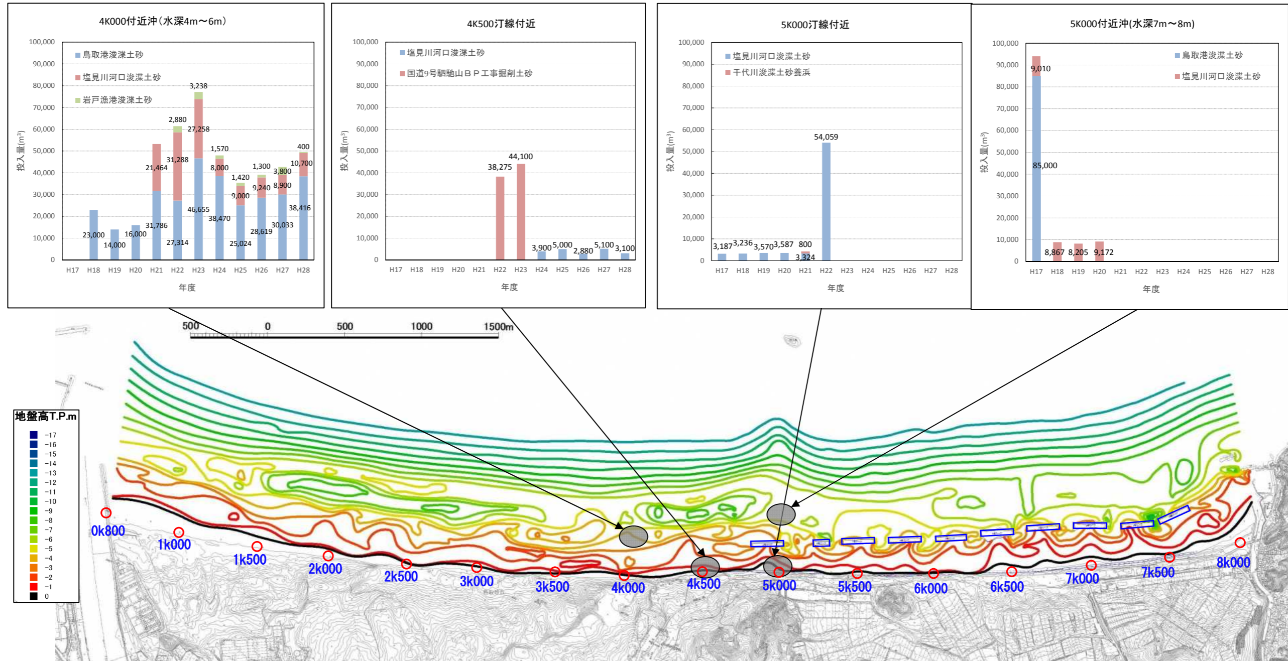
図 4.2.2 鳥取砂丘前面の土砂投入実績(等深線図 H29.3 測量)
