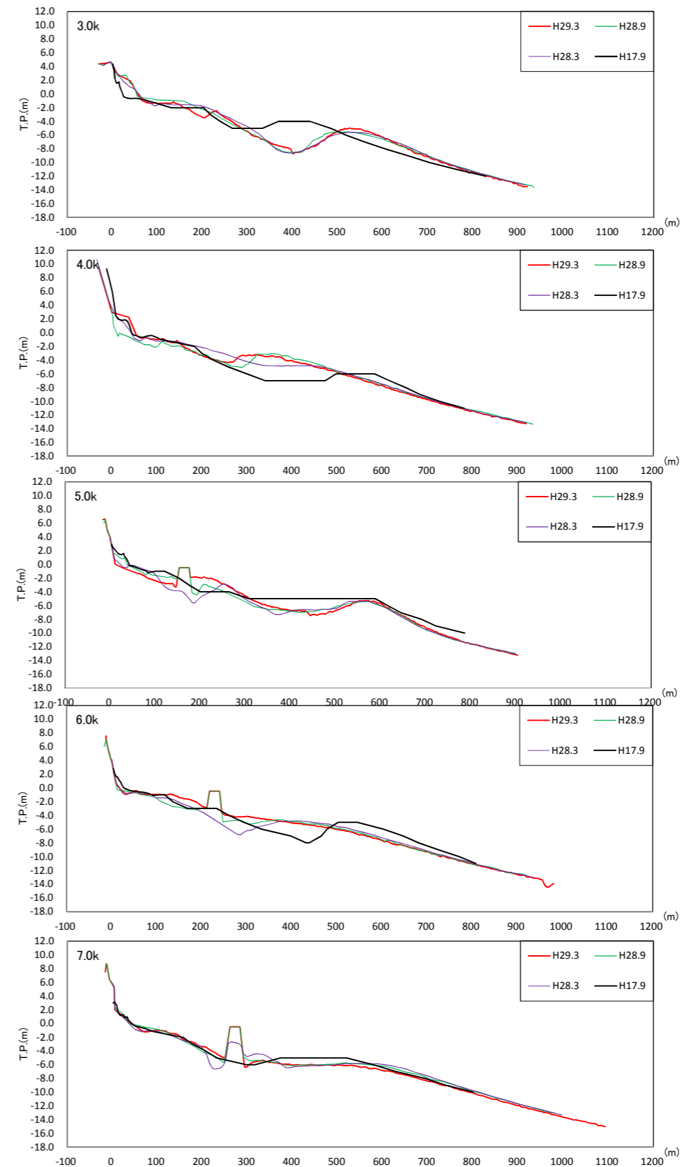
図 4.3.10 湯山海岸の横断変化図（平成 17 年 9 月～平成 29 年 3 月）(2)
