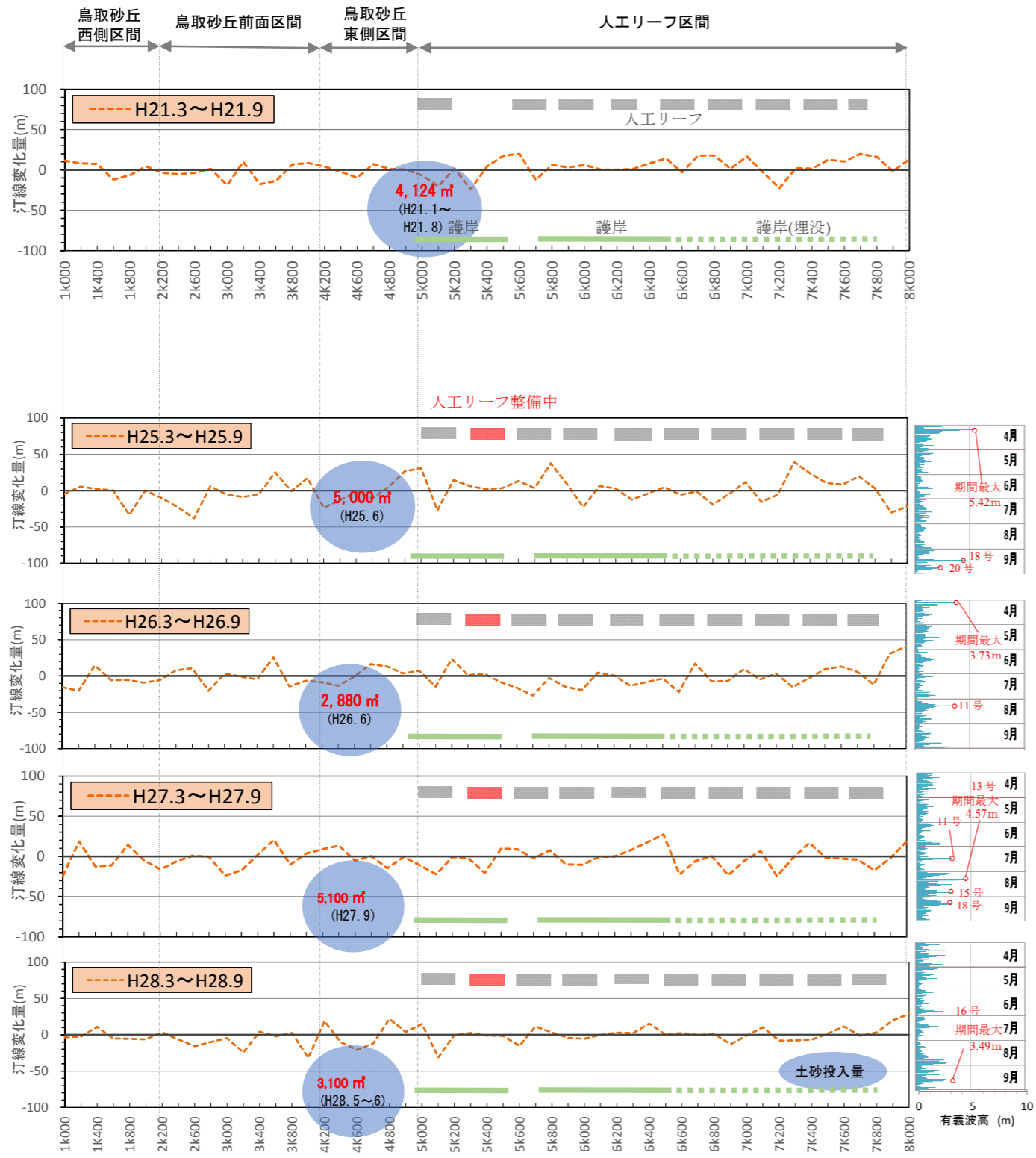
図 4.3.6 サンドリサイクル開始以後の汀線変化状況図
