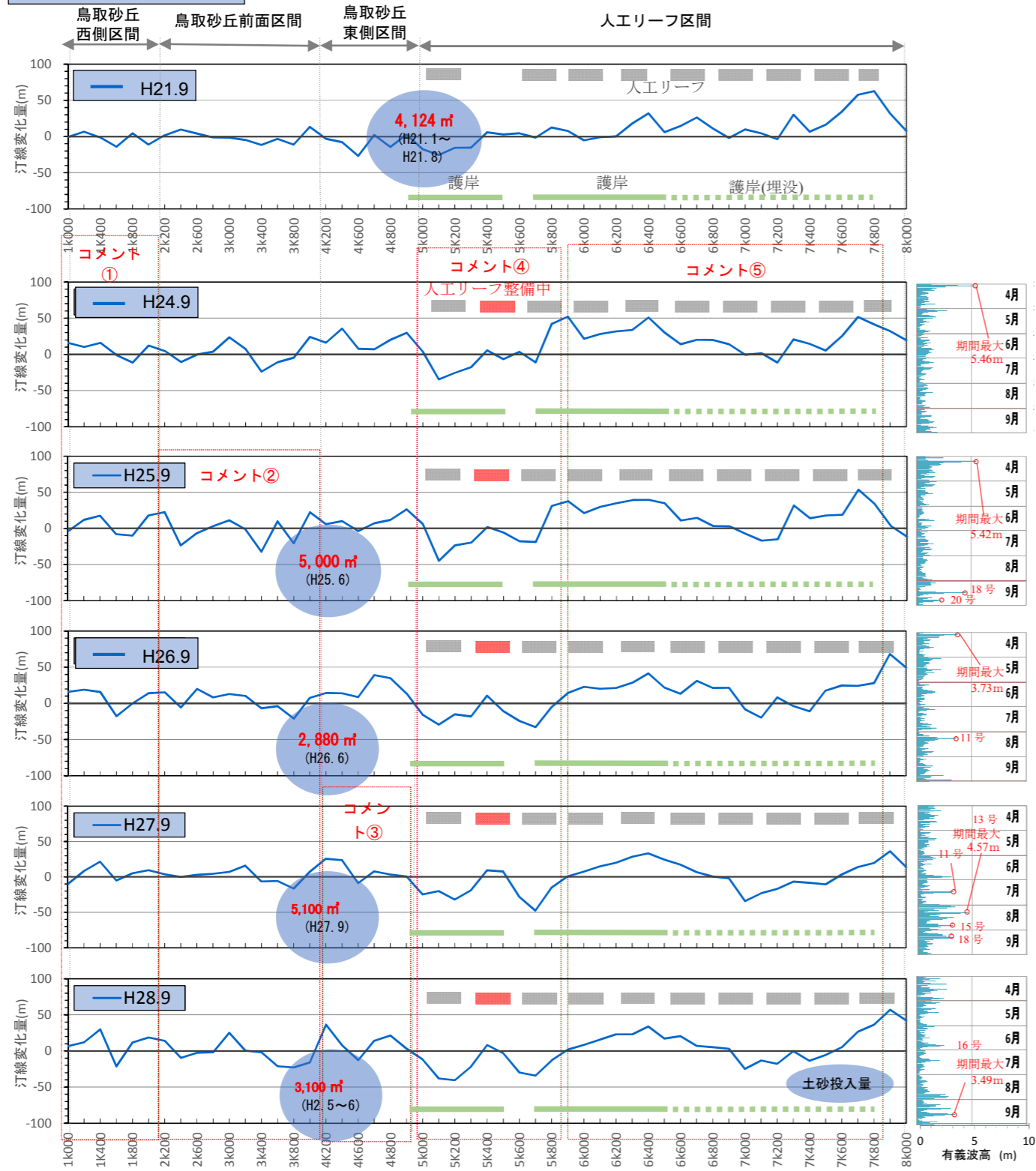
図 4.3.4 サンドリサイクル開始以後の汀線変化状況図(平成 18 年 9 月基準)
