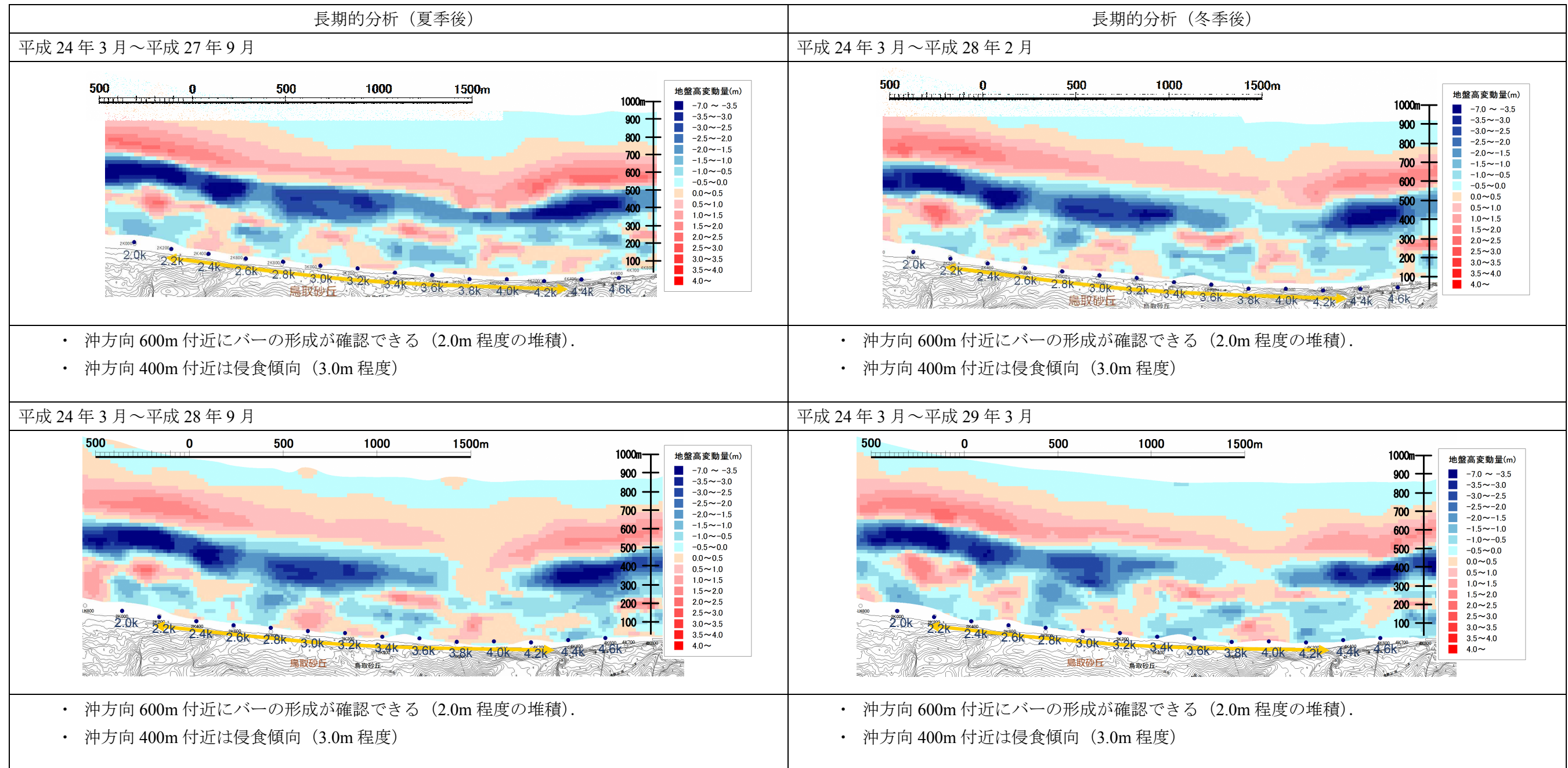
図 4.3.12 標高差分図(平成 24 年 3 月を基準とした長期的分析)
