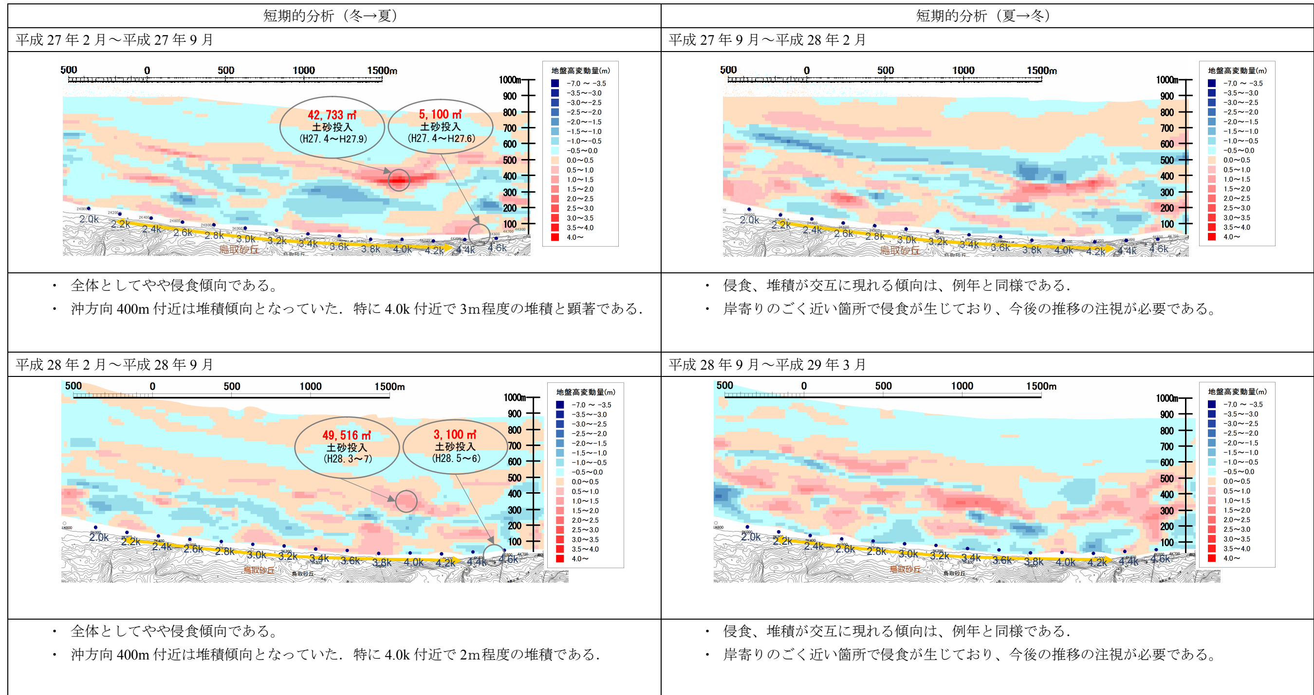
図 4.3.14 標高差分図（短期的分析）
