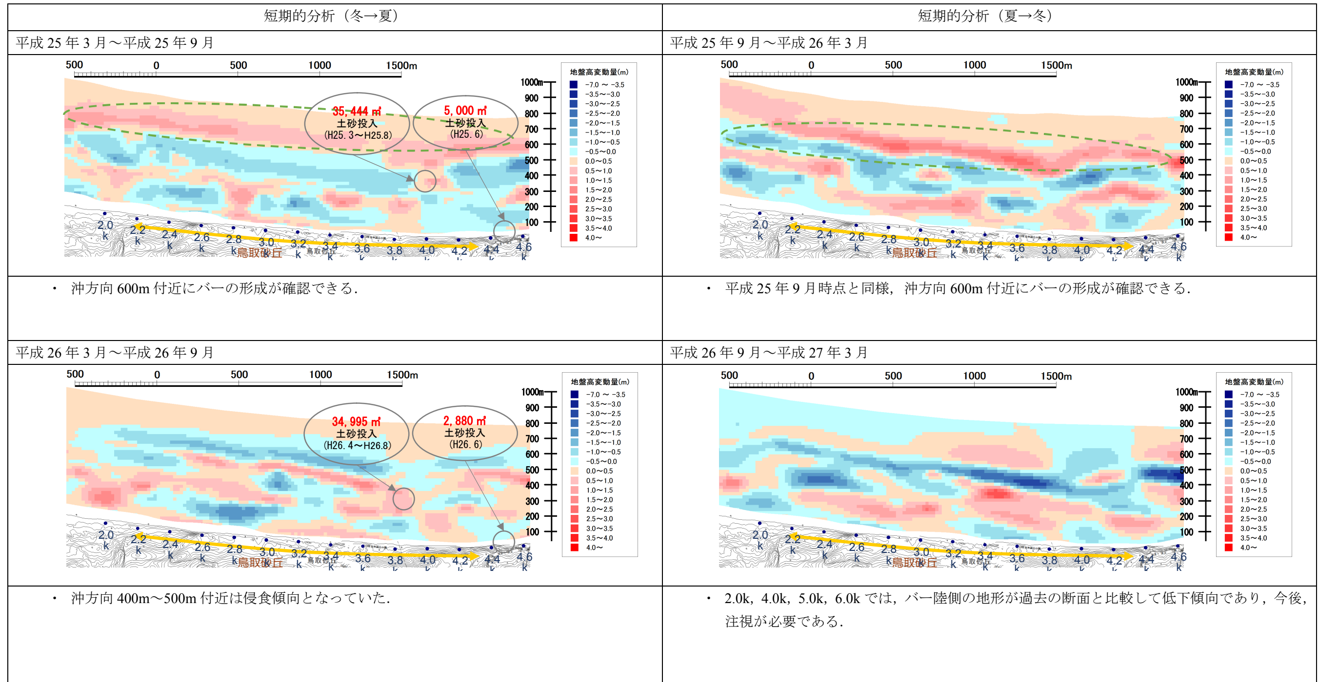
図 4.3.13 標高差分図（短期的分析）
