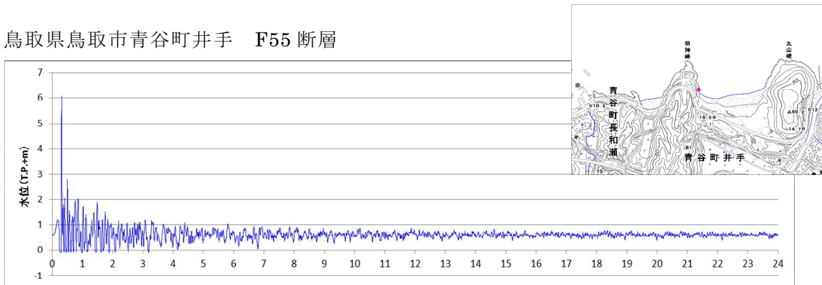
図-9 主な地点での水位変化
