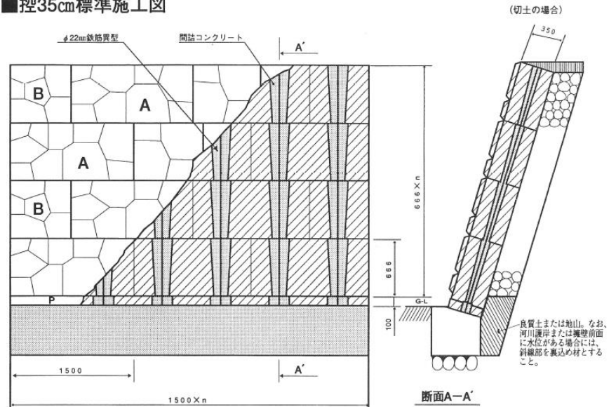
■控35cm標準施工図
