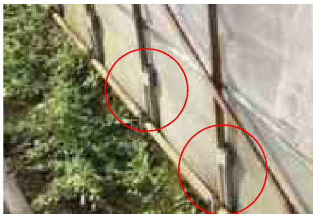
写真 パイプハウスの地際部補強(○枠)の例
