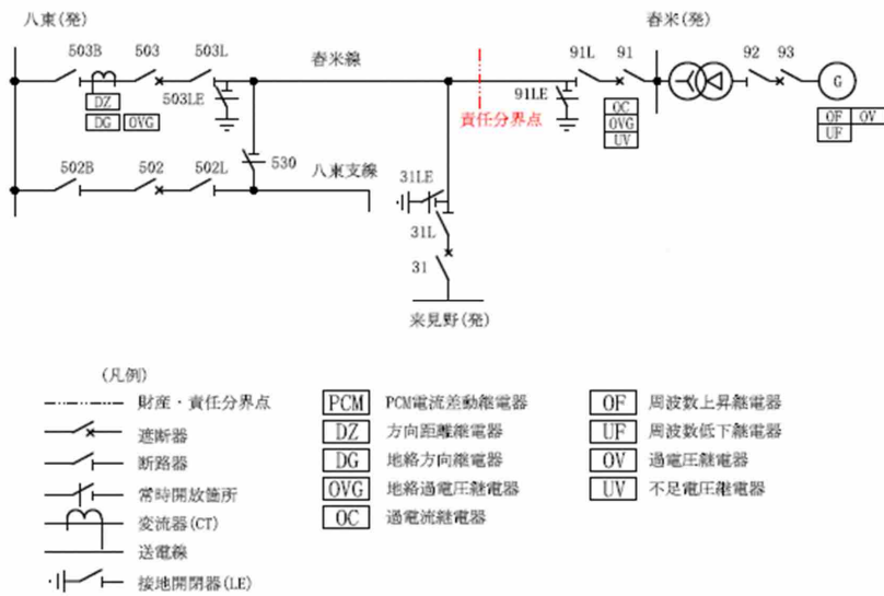
図-2 責任分界点（春米発電所）
