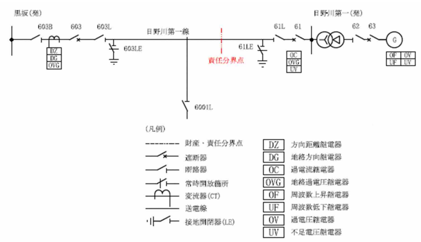
図-3 責任分界点 (日野川第一発電所)
