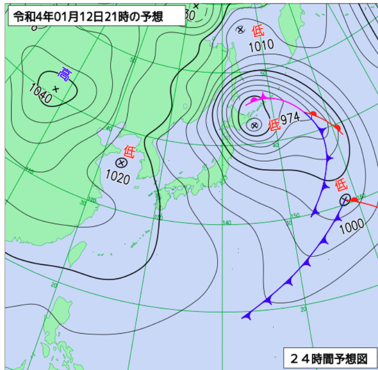
12日21時予想図
