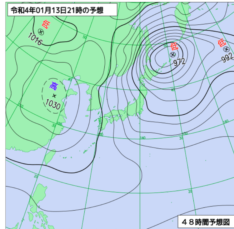
13日21時予想図
