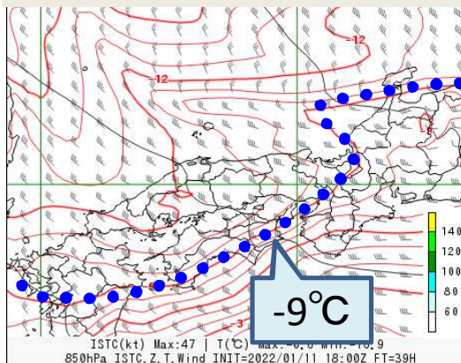
約1500m 気温
