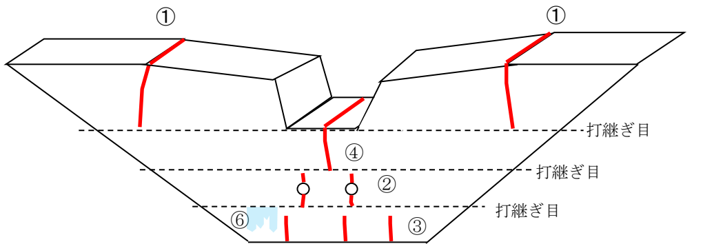
(a) 打継ぎ目から鉛直方向に進展するひび割れや断面急変部、欠損部などに見られるひび割れ
