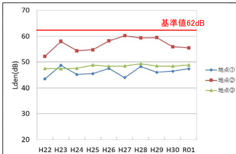
騒音調査の結果(環境省の新基準値:Lden)
