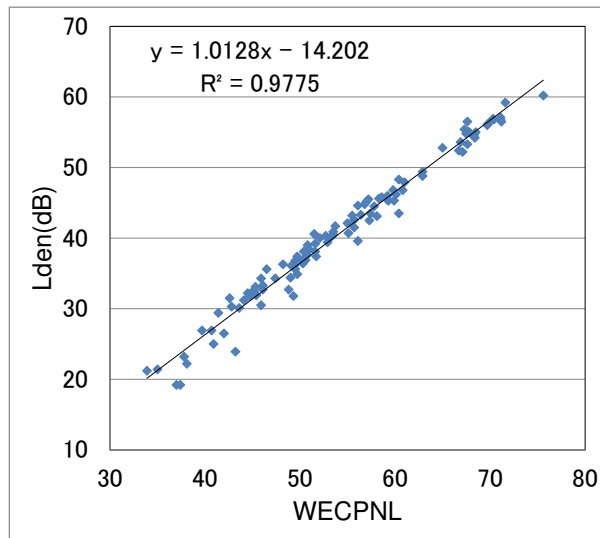
図4 Lden と WECPNL との相関(N=108)
