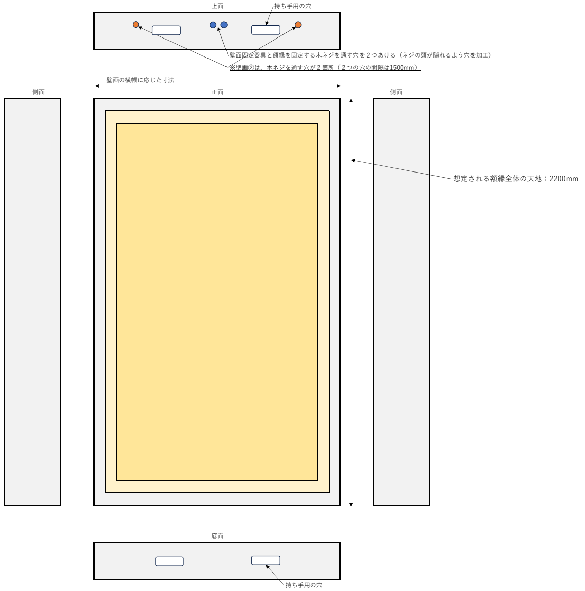
額縁Bタイプの基本構造図（上面、側面、正面図）
