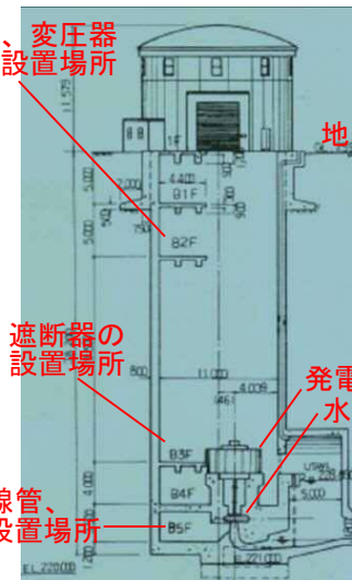
<発電所断面図>
