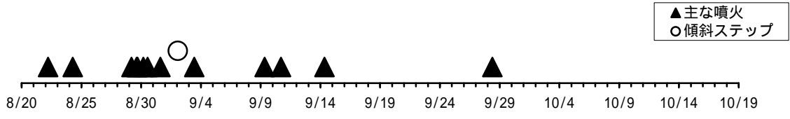
図3 三宅島の火山活動経過図 (2000年8月20日~10月18日)
