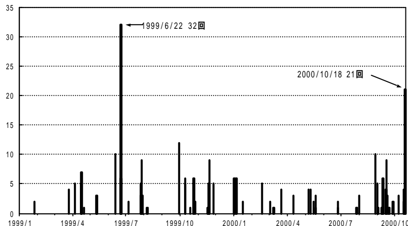
図2 富士山の日別の低周波地震回数 (1999年1月1日~2000年10月18日)
