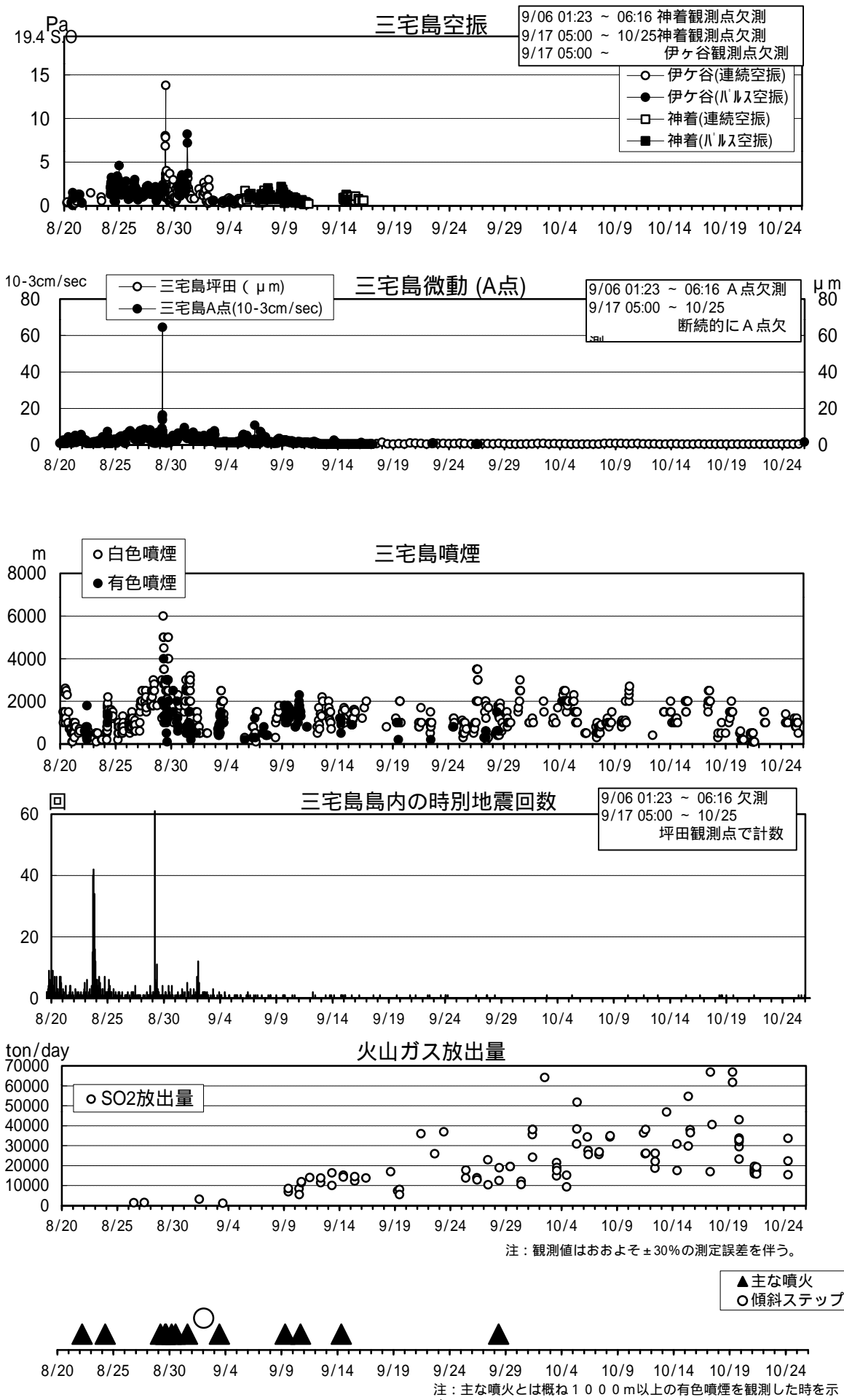
図2 三宅島の火山活動経過図 (2000年8月20日~10月25日) 測候所観測点は神着観測点と名称を変更した。
