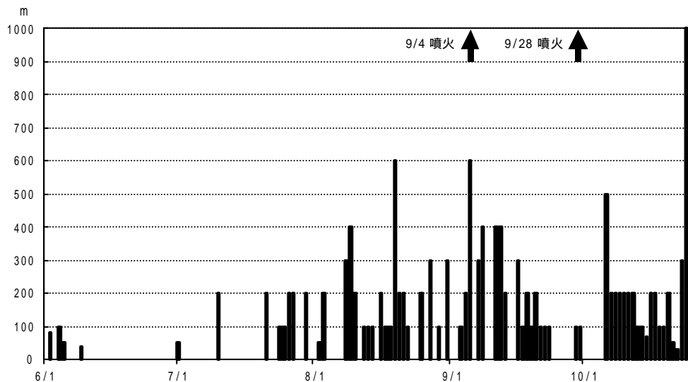
図1 北海道駒ヶ岳の日別最大噴煙の高さ（2000年6月1日～10月25日）
