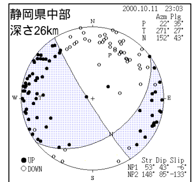
P波初動による 下半球投影
