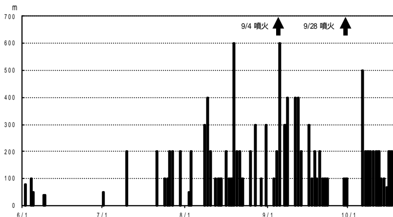
図1 北海道駒ヶ岳の日別最大噴煙の高さ (2000年6月1日~10月18日)
