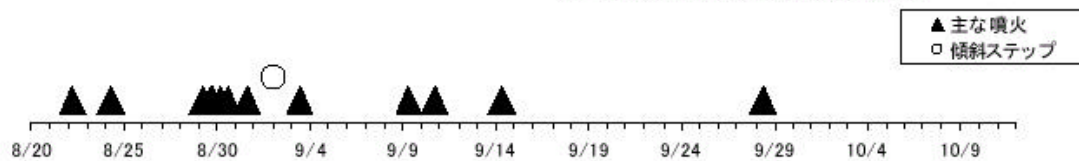
図2 三宅島の火山活動経過図 (2000年8月20日~10月11日)
