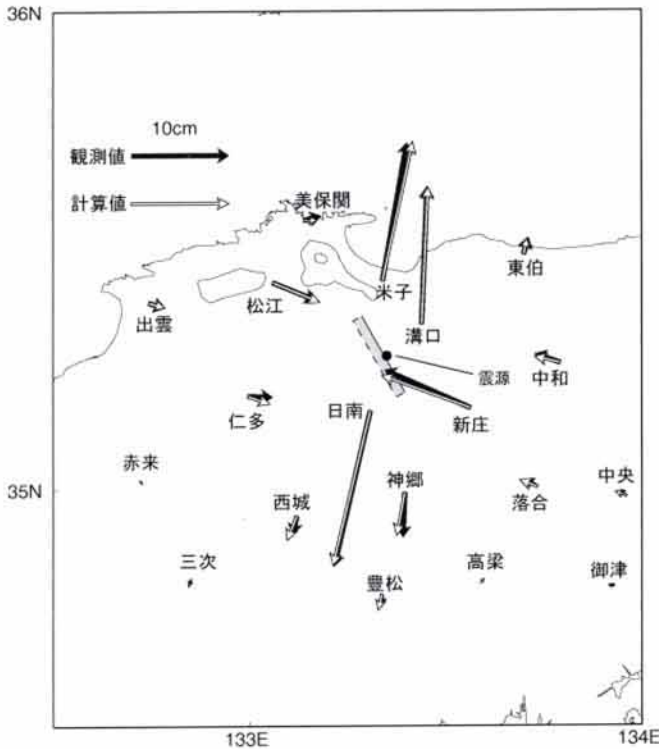
平成12年10月6日鳥取県西部地震に伴う地殻変動と断層モデル
