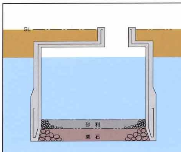
井戸式防火水槽
