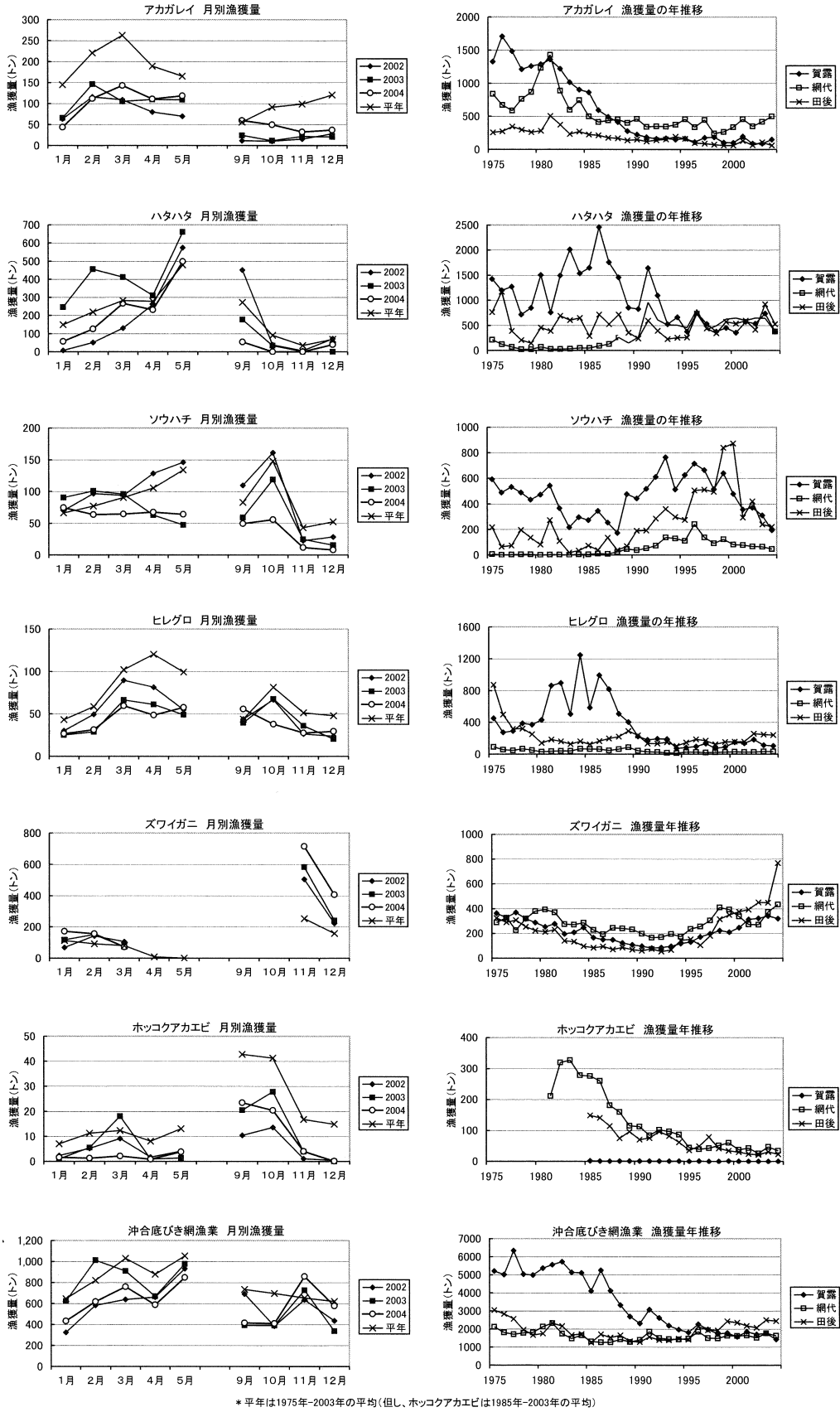
図2 鳥取県沖合底びき網漁業主要魚種の月別漁獲量及び漁獲量の年推移
