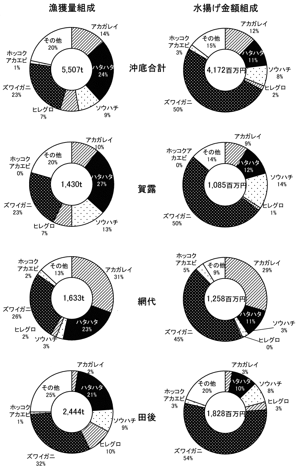
図1 鳥取県沖合底びき網の漁獲量及び水揚げ金額の組成 (2004年)
