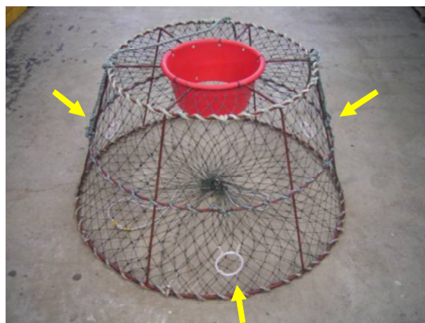
図7 試験籠写真 (13cm目合リング(内径95mm脱出口3個)付き)
