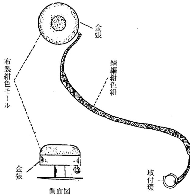
平面図
