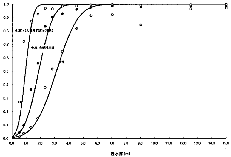
図 5.1-2 建物被害と浸水深の関係（上段：木造／下段：非木造）
