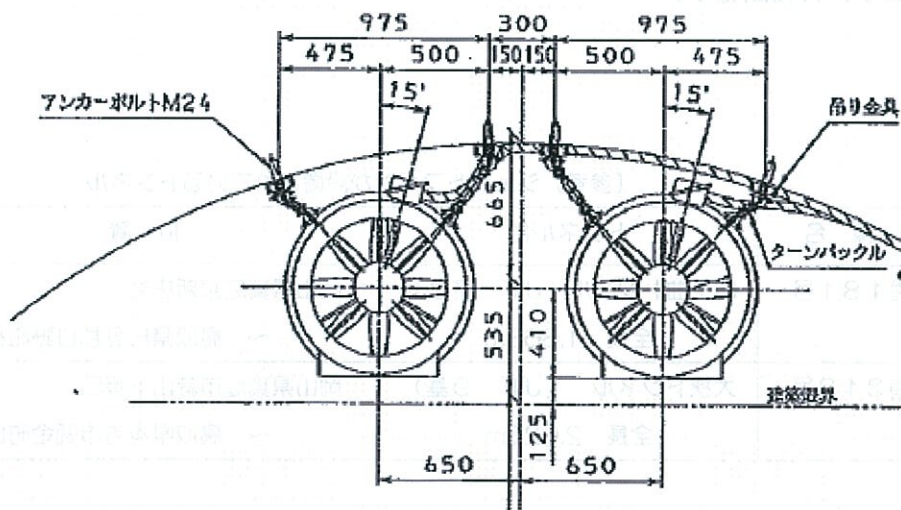
【構造図】
