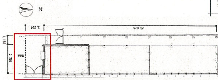
物置き及び薪小屋平面図
