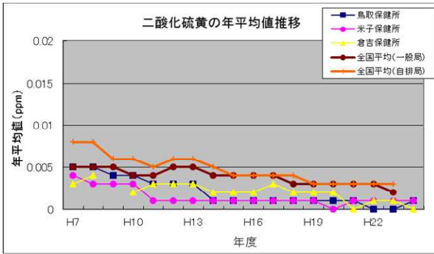
図 5-1 二酸化硫黄
