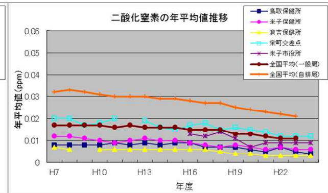
図 5-4 二酸化窒素
