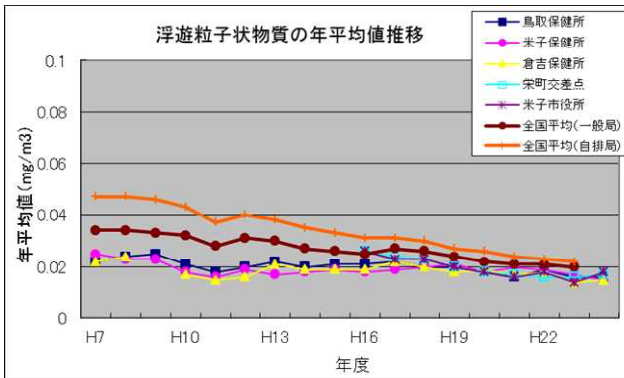
図 5-3 浮遊粒子状物質
