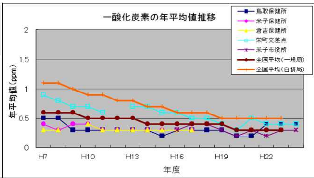
図 5-2 一酸化炭素
