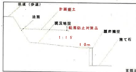
計画横断面図
