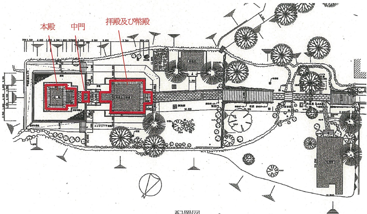
配置図
