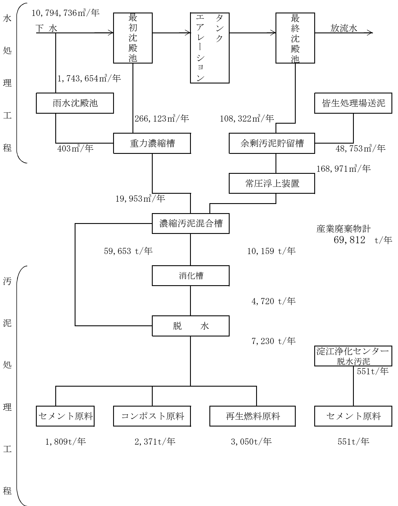
水処理・汚泥処理フローシート
