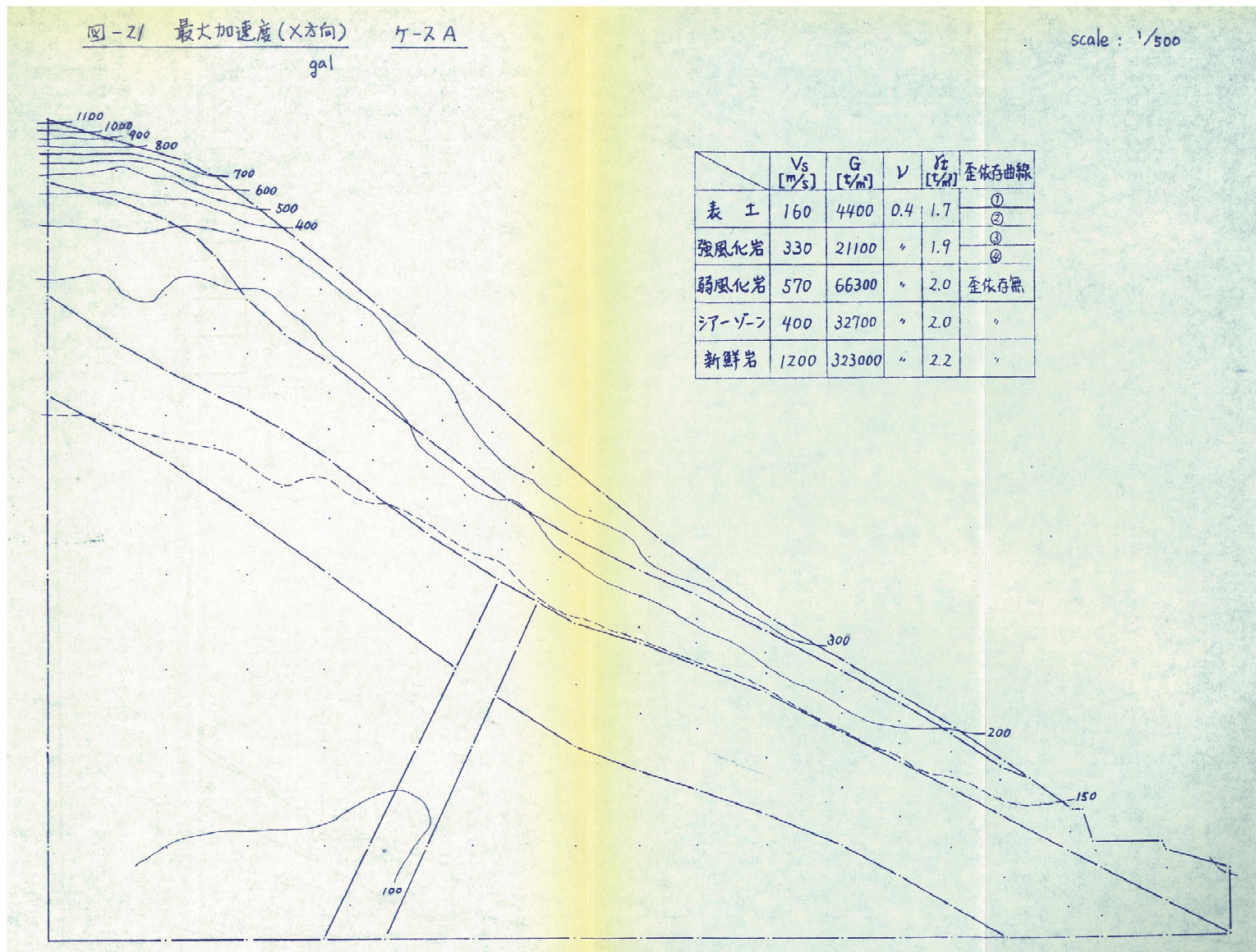
図 1.1-2(2) 1978年伊豆大島近海地震の際の崩壊斜面の解析(1980) 最大水平加速度分布図
