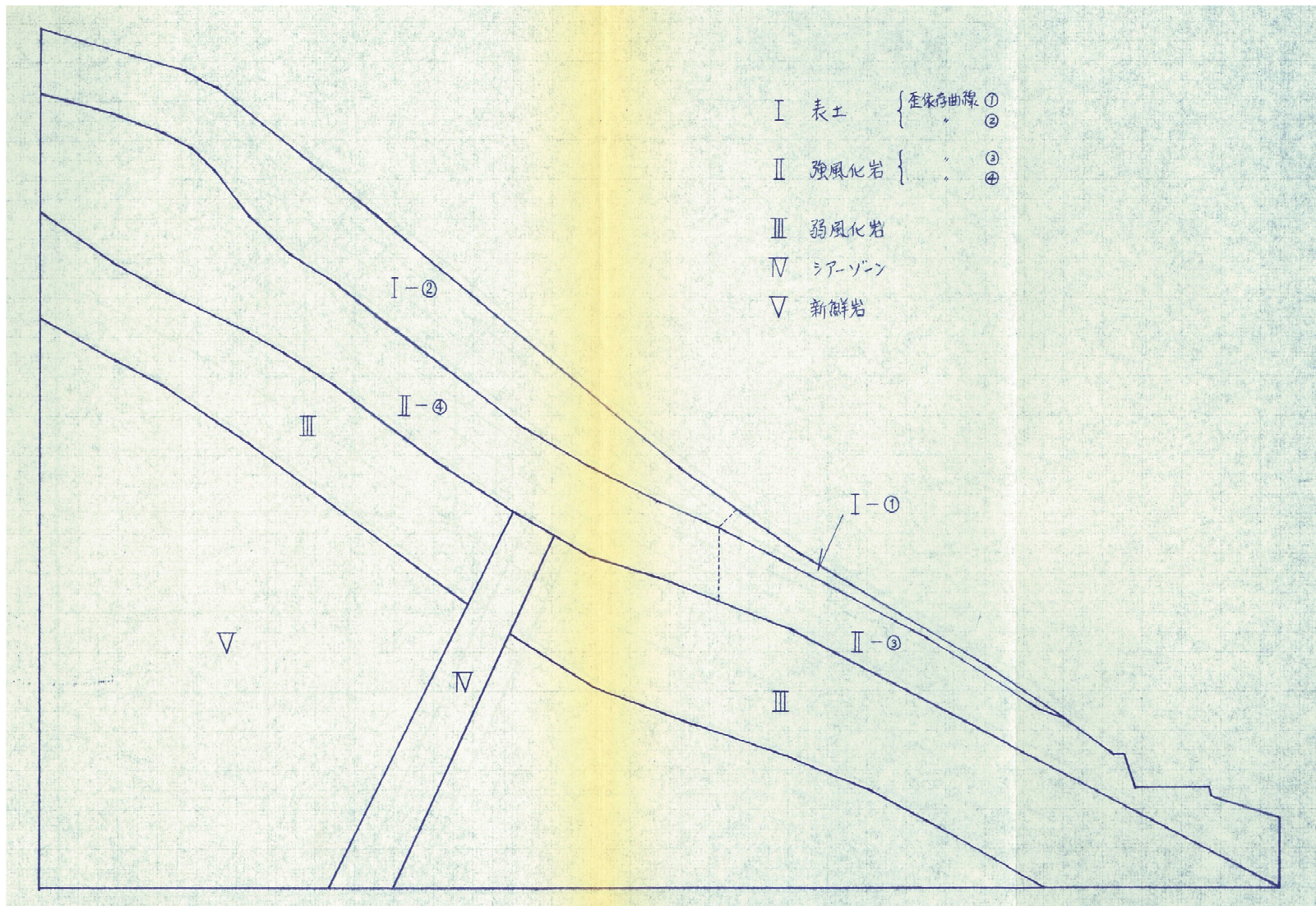
図 1.1-2(1) 1978 年伊豆大島近海地震の際の崩壊斜面の解析(1980) 物性区分図
