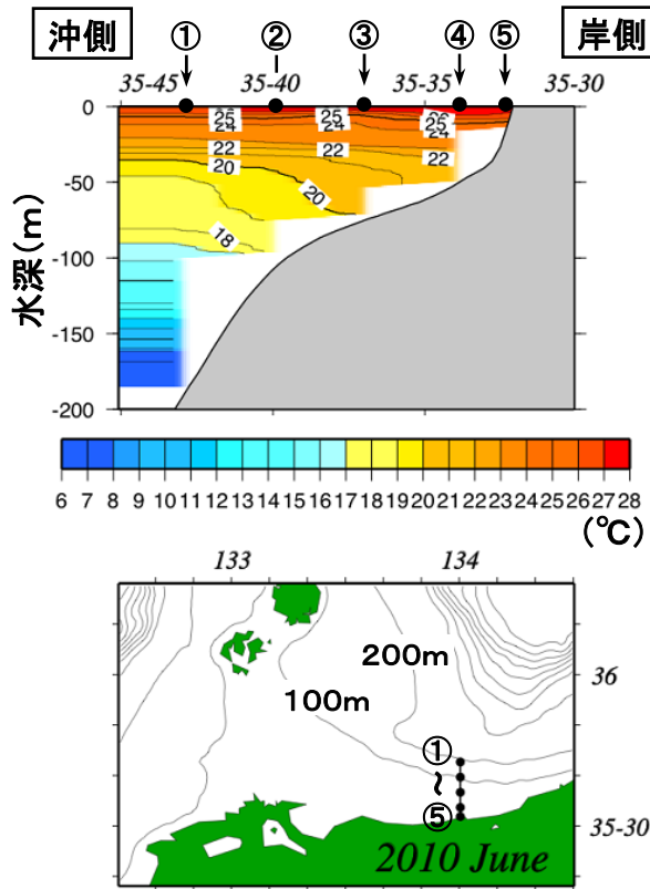
図1) 7月22日の水温の鉛直断面図
