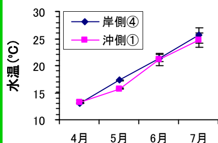
図2) 4～7月の20m以浅の水温の平均値の季節変化。
