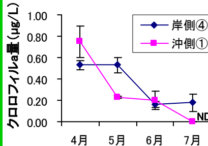
図3) 4～7月の20m以浅のクロロフィルaの平均値の変化。ND: 検出限界以下。
