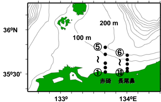
図1) H24年11月30日の調査地点(左)と赤碕(中央)と長尾鼻(右)地先における水温の鉛直分布
