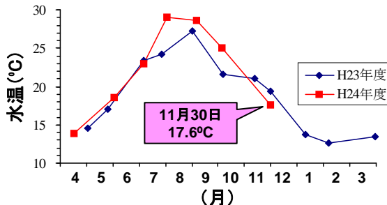
図2) 長尾鼻地先の水深50 m地点(⑨)における海面水温の季節変化。
