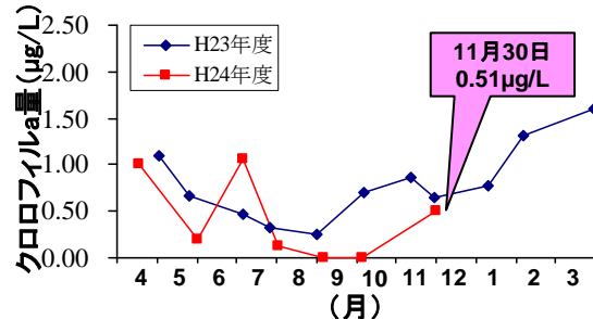
図3) 長尾鼻地先の水深50 m地点(⑨)における表層クロロフィルa量の平均値の季節変化。
